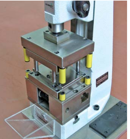
超薄フィルム抜型
