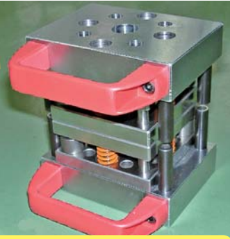
加圧成形型
